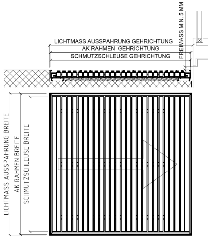
Variante: versenkte Matte
