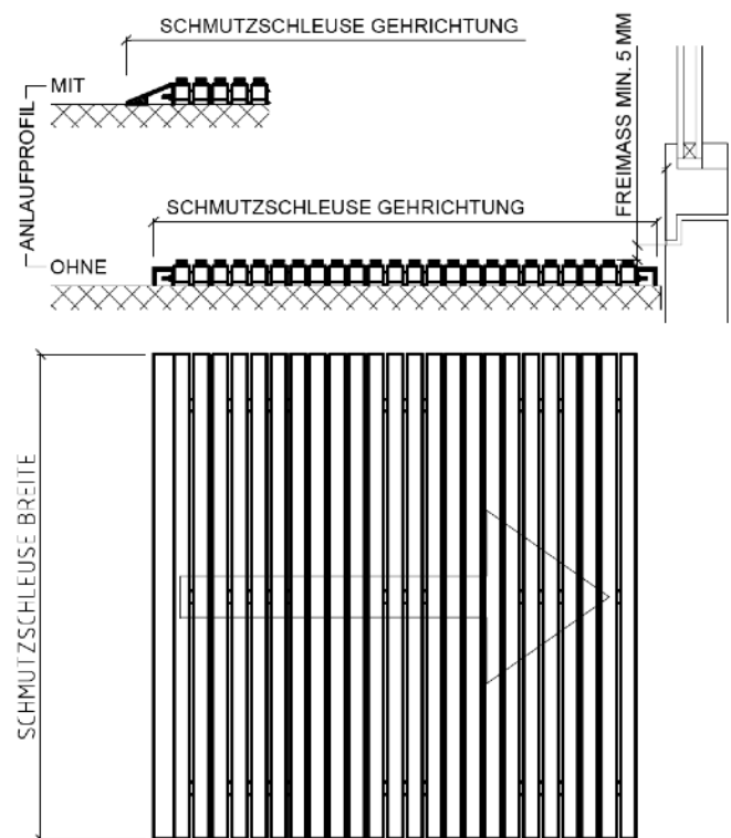
Variante: aufgelegte Matte
